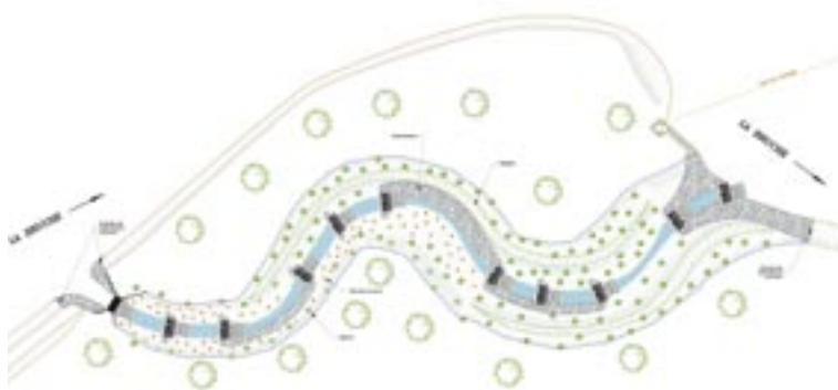
Schéma de la rivière artificielle de contournement (110 mètres).
